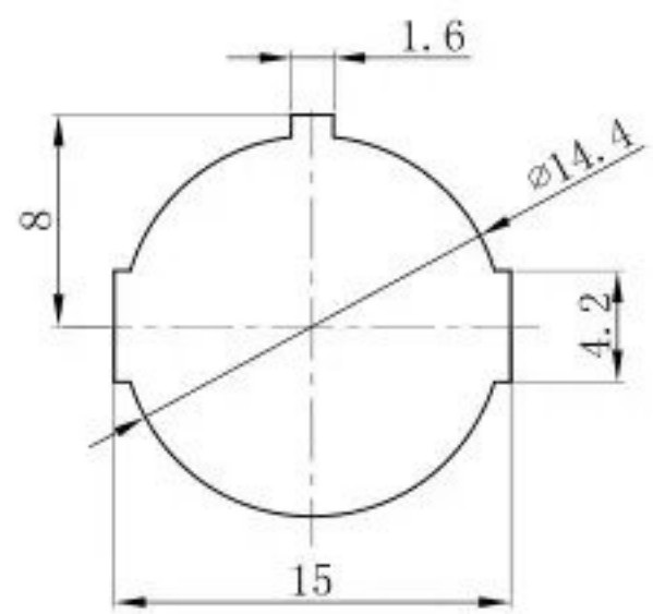
安装面板尺寸 PANEL CUT-OUT
