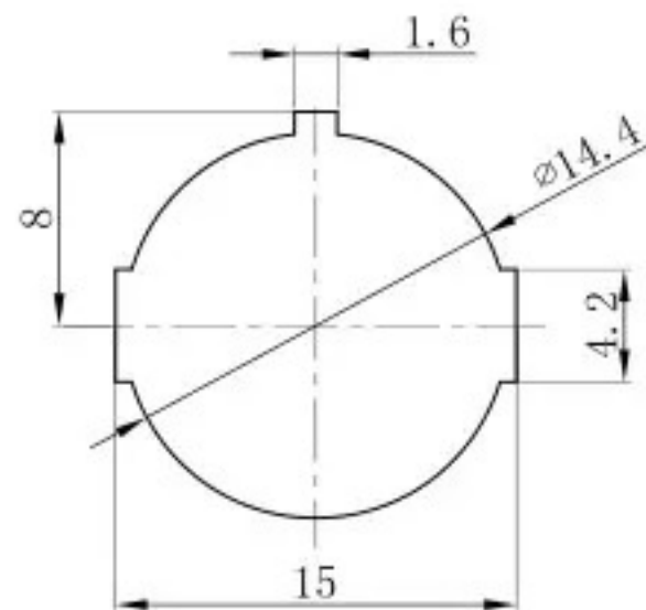
安装面板尺寸 PANEL CUT-OUT
