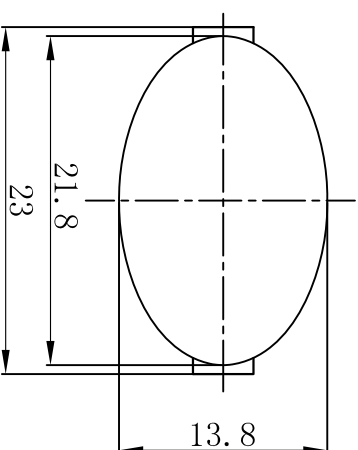
安装面板尺寸 PANEL CUT-OUT
