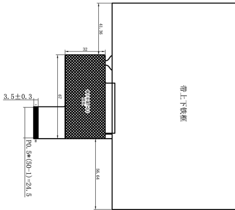
背视图
