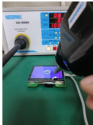
3.1 静电放电测试图
