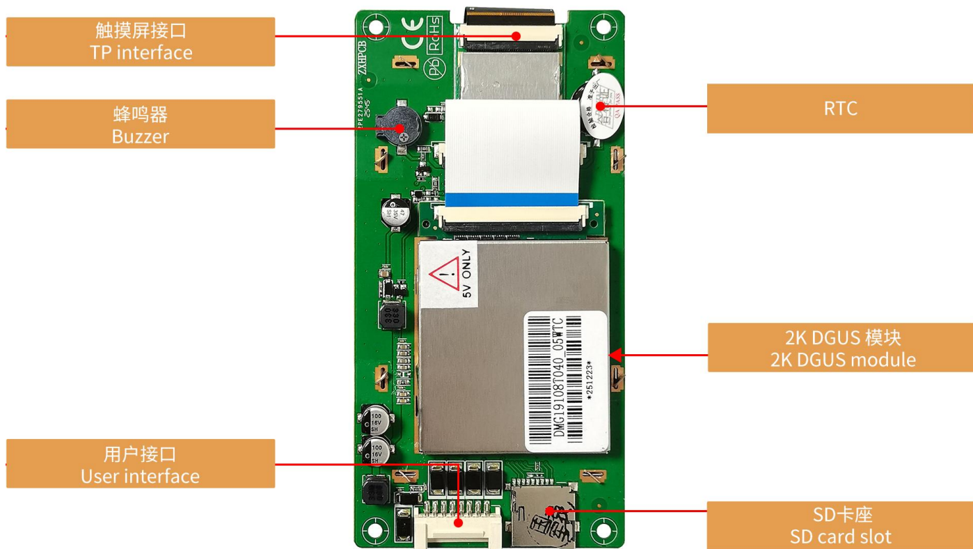
硬件接口图
