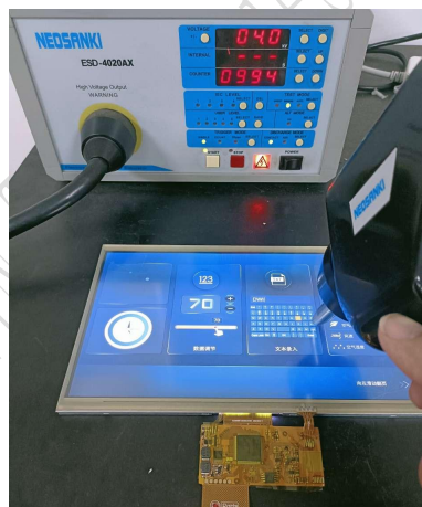
4.1 静电放电测试图
