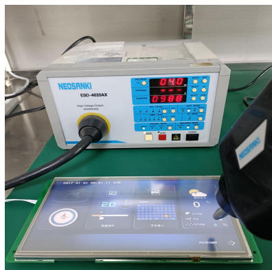
3.1 静电放电测试图 Electrostatic discharge test
