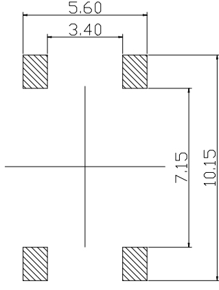
PCB. 焊接图
