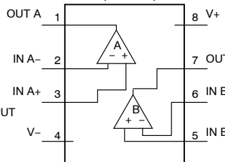
UDFN8/Micro8/SOIC-8
